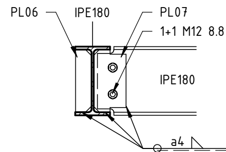
BALK-BALKKOPPLING 1 : 10
